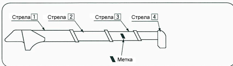
● 4-х секционная стрела
