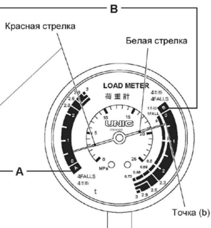
Рис. 2 Индикатор грузоподъемности
