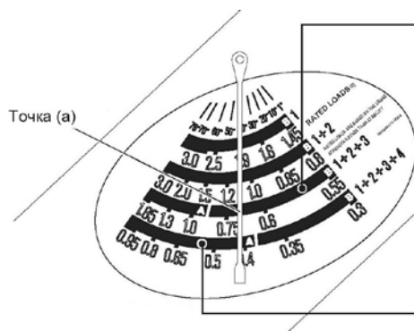
Рис. 1 Указатель грузоподъемности (на примере КМУ URV294)
